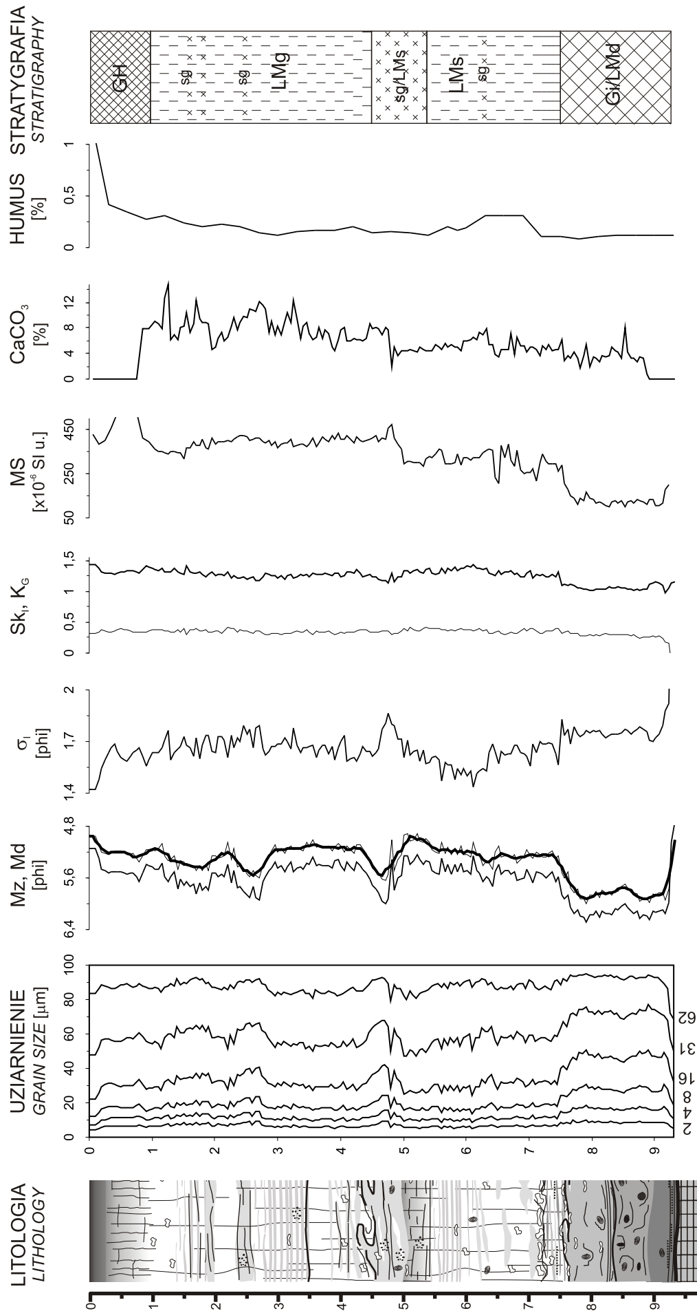
Ryc. 17. Profil górnopleistocénskich lessów i gleb kopalnych w Księginicach Małych. Md wg Inmana (1952); Mz, \delta , Sk 1 , K G wg Folka i Warda (1957); MS - podatność magnetyczna. Objaśnienia sygnatur litologicznych i stratygraficznych jak na rycinie 9 Fig. 17. Upper Pleistocene loess section at Księginice Małe. Md acc. to Inman (1952); Mz, \delta , Sk 1 , K G acc. to Folk and Ward (1957); MS - magnetic susceptibility. Explanations of lithologic and stratigraphic signatures as in figure 9
