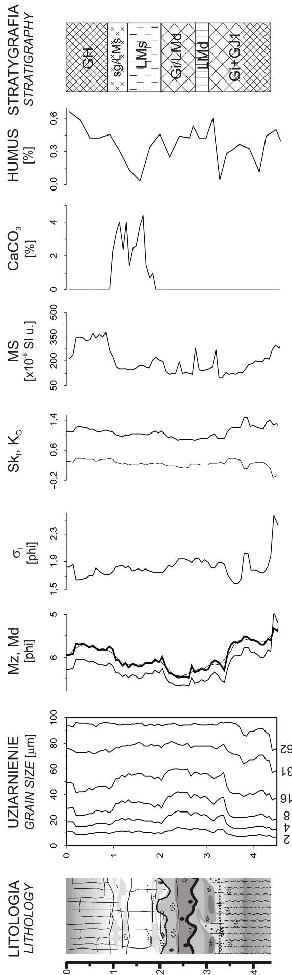
Ryc. 20. Profil górnopleistocenów i gleb kopalnych w Branicach. Md wg Inmana (1952); Mz, \delta_i , S_k , K_G wg Folk i Warda (1957); MS - podatność magnetyczna. Objasnienia sygnatur litologicznych i stratygraficznych jak na rycinie 9
