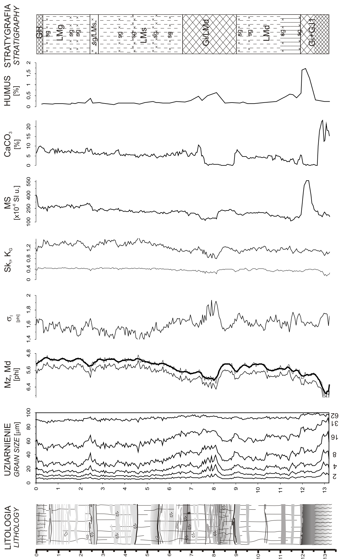
Ryc. 10. Profil górnoplejstocénskich lessów i gleb kopalnych w Polanowie Samborzeckim k. Sandomierza. Md wg Inmana (1952); Mz, \delta_p , Sk p , K c wg Folk i Warda (1957); MS - podatność magnetyczna. Objaśnienia sygnatur litologicznych i stratygraficznych jak na rycinie 9
