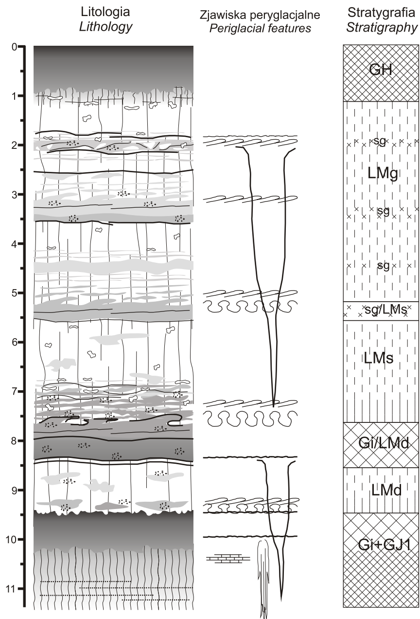
Ryc. 33. Zjawiska peryglacjalne, litologia i stratygrafia w profilu Korshov. Objaśnienia sygnatur litologicznych i stratygraficznych jak na ryc. 9. Objaśnienia zjawisk peryglacjalnych jak na ryc. 26
