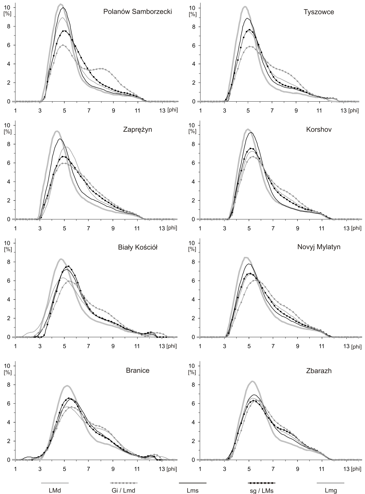
Ryc. 23. Reprezentatywne krzywe częstości uziarnienia jednostek litostratigraficznych lessów młodszych w wybranych stanowiskach
