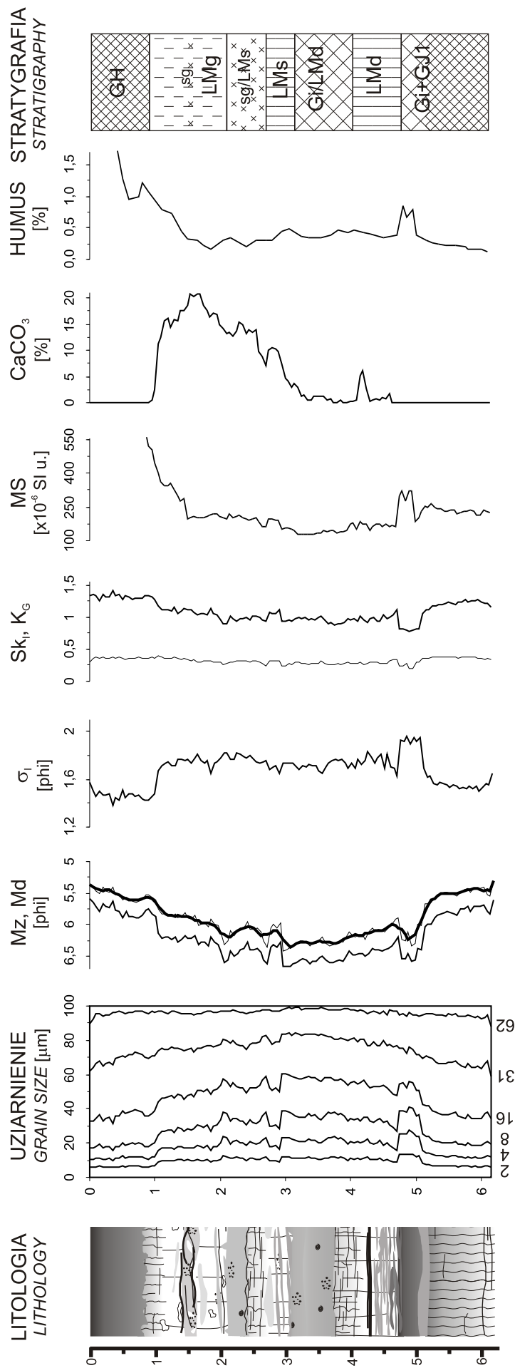
Ryc. 19. Profil górnoplejstocénskich lessów i gleb kopalnych Zbarazh. Md wg Inmana (1952); Mz, \delta_i , S_{k_i} , K_G wg Folka i Warda (1957); MS - podatność magnetyczna. Objasnienia sygnatur litologicznych i stratygraficznych jak na rycinie 9 Fig. 19. Upper Pleistocene loess section at Zbarazh. Md acc. to Inman (1952); Mz, \delta_i , S_{k_i} , K_G acc. to Folk and Ward (1957); MS - magnetic susceptibility. Explanations of lithologic and stratigraphic signatures as in figure 9
