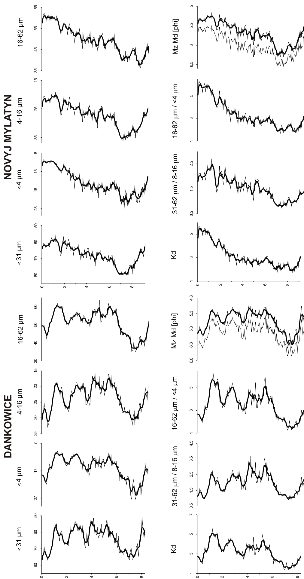
Ryc. 21. Zmiany różnych wskaźników uziarnienia dla górnoplejstocенских sekwencji lessów i gleb kopalnych na stanowisku Dankowice i Nowy Mylatyn, przedstawione jako funkcja głębokości
