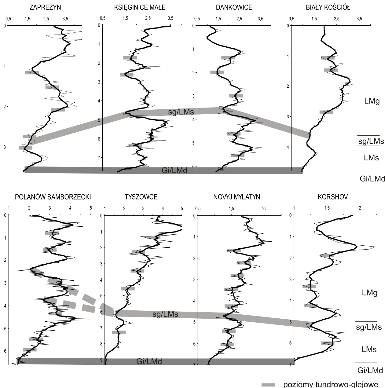
Ryc. 24. Stosunek frakcji grubego (31-62 μm) do drobnego (8-16 μm) pyłu dla sekwencji lessów młodszych zalegających ponad stropem gleby Gi/LMd (komorniki). Ciągłą linią połączono strop gleby Gi/LMd oraz poziom sg/LMs, a poziomy tundrowo-glejowe w lessach młodszych górnych i środkowych zaznaczono szarymi znacznikami
